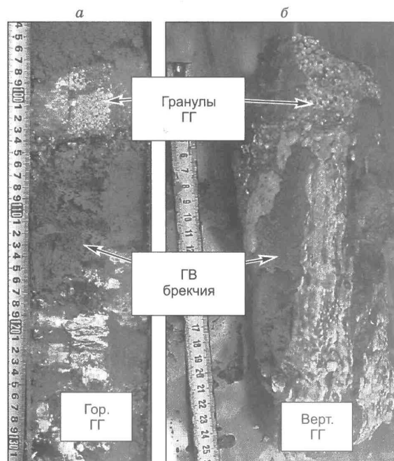
Рис. 2. Фотографии участков керна со слоями газовых гидратов в виде гранул.
