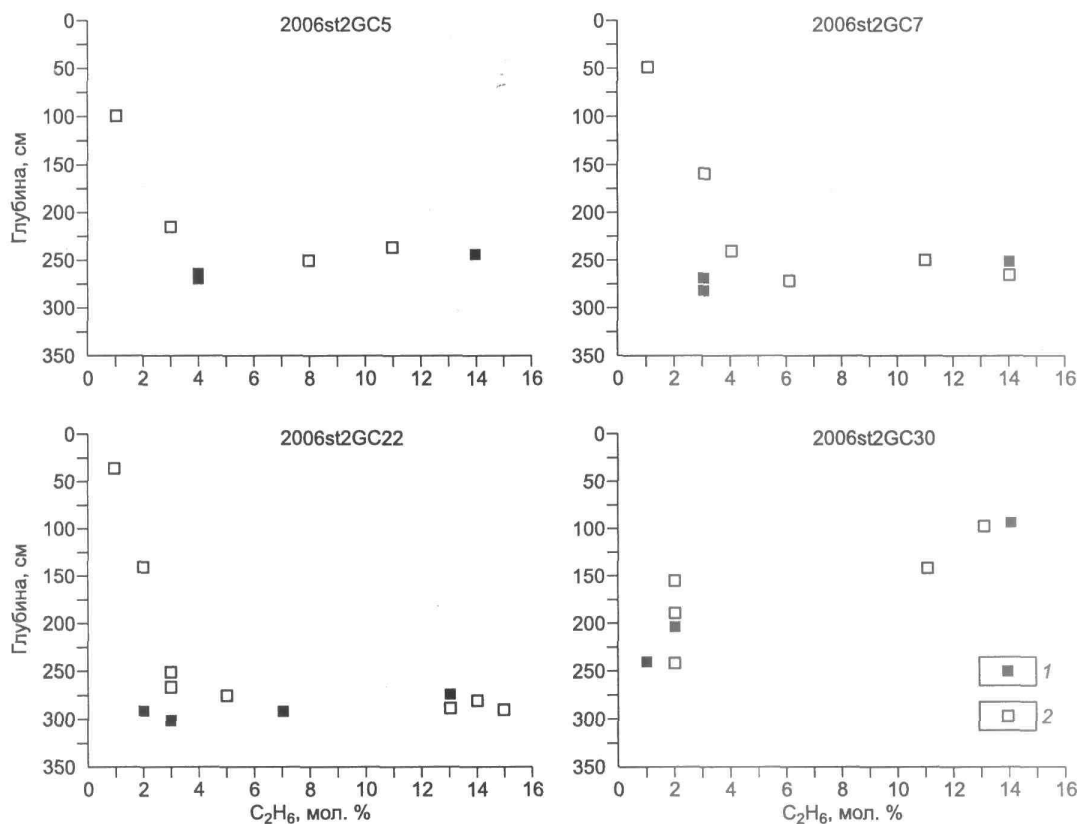
Рис. 5. Концентрации этана в газовом гидрате (1) и в растворенном газе (2) в зависимости от глубины для кернов, отобранных на грязевом вулкане К-2 [Nachikubo et al., 2010].
