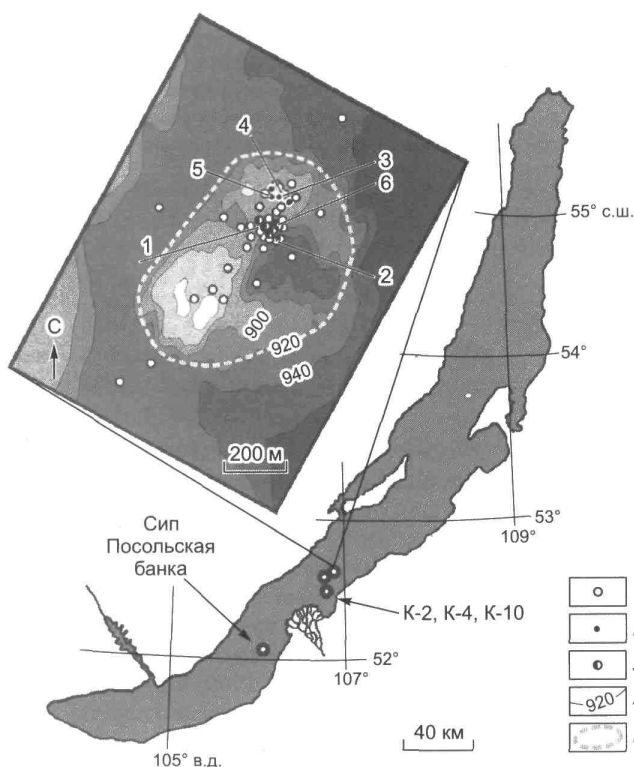
Рис. 1. Структура грязевого вулкана К-2.
