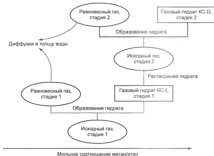
Рис. 3. Схема, иллюстрирующая образование гидрата КС-II.
